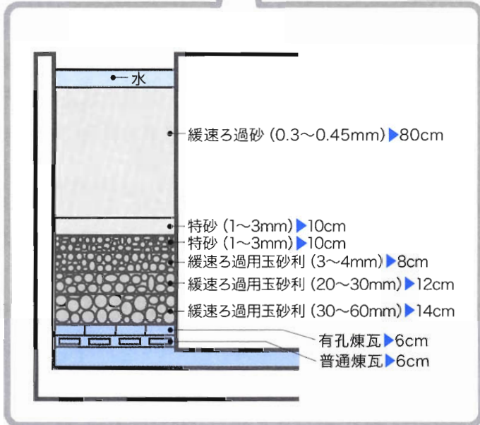
ろ過池の断面図
